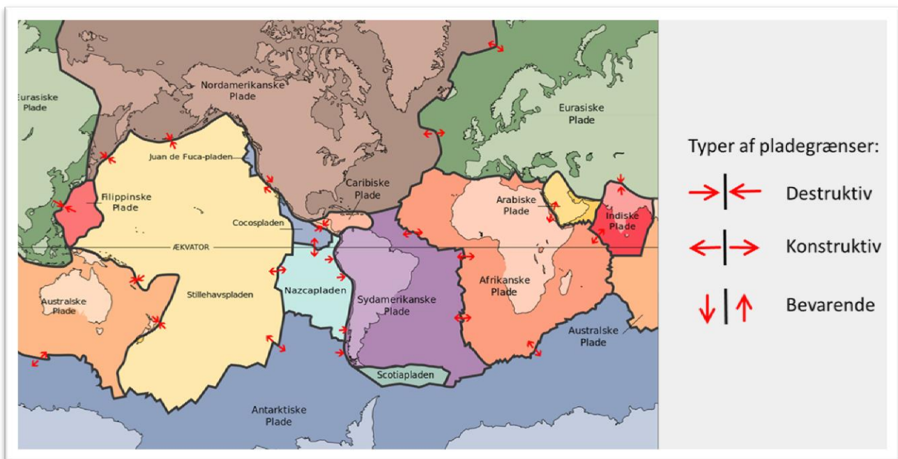
Figur 2 - De tektoniske plader
